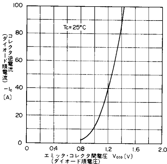
コレクタ逆電流 順電流 -I_c (A) エミッタ・コレクタ間電圧 V_{cco} (V) (ダイオード順電圧) 高速フリーホイリングダイオード順電圧 Forward Voltage of Free Wheeling Diode
