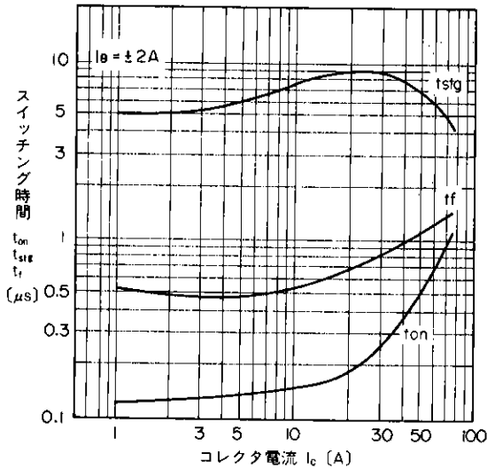
スイッチング時間 I_b = \pm 2A コレクタ電流 I_c (A) スイッチング時間—コレクタ電流特性 Switching Time
