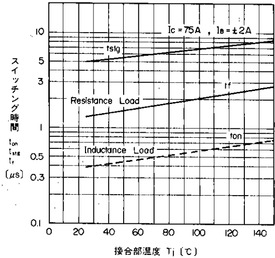
スイッチング時間 I_c = 75A, I_b = \pm 2A 接合部温度 T_j (°C) スイッチング時間—接合温度特性 Switching Time
