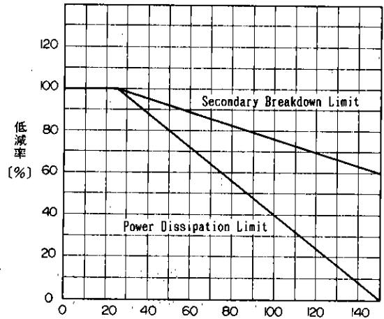
ケース温度 T_c (°C) ASO 低減特性 ASO Derating
